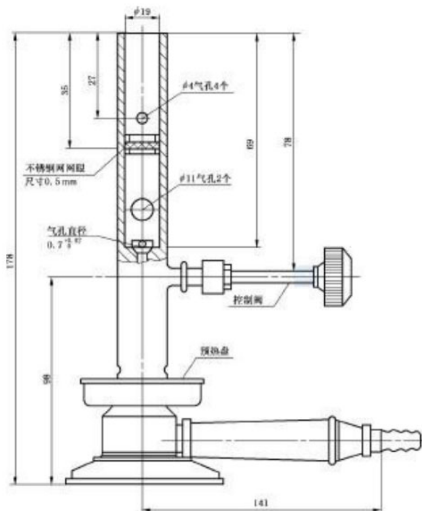
图 5 酒精喷灯
