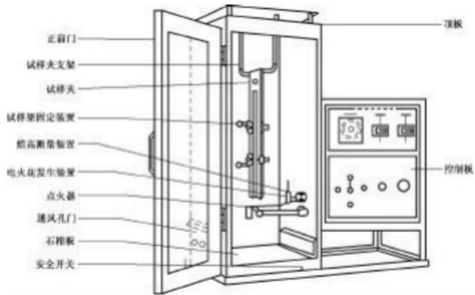
图 1 燃烧试验箱构造图
