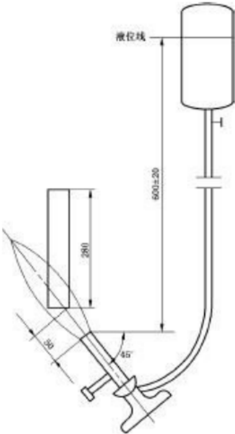
图 4 酒精喷灯试验装置
